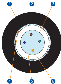
4,8&12 Fibre Construction
